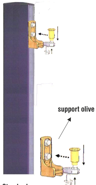
Poteau de guidage
